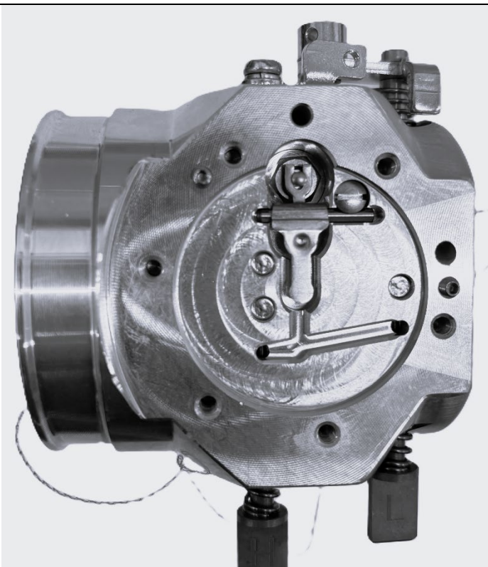
Photo côté aspiration (vue additionnelle) / Photo of inlet side (additional view)
